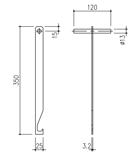
オプション：開閉フック (MF-62) (S45C) 電気亜鉛めっき
