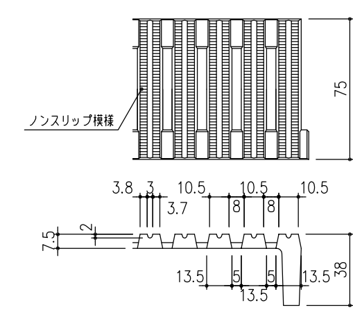
ノンスリップ詳細図 S=1/2
