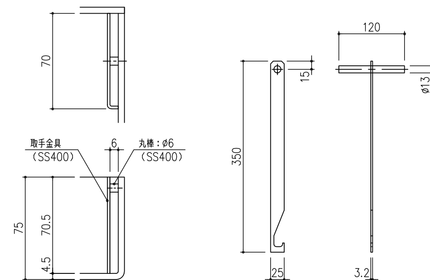
取手金具 詳細図 S=1/2
