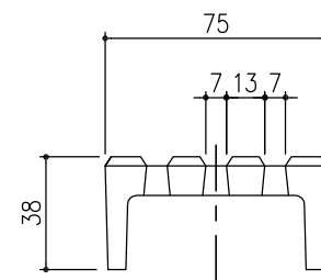
スレンダー側溝蓋 詳細図 S=1/2
