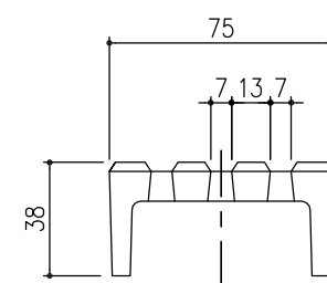
スレンダー側溝蓋 詳細図 S=1/2
