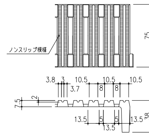
ノンスリップ詳細図 S=1/2
