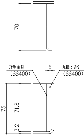
取手金具 詳細図 S=1/2
