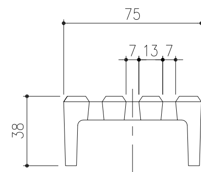
スレンダー側溝蓋 詳細図 S=1/2
