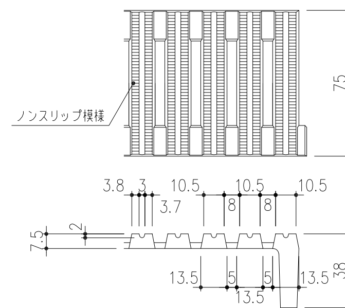
ノンスリップ詳細図 S=1/2
