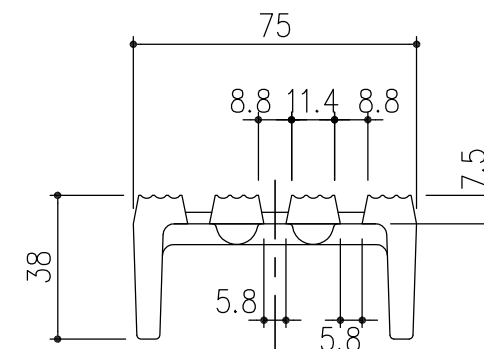
ノンスリップ詳細図 S=1/2
