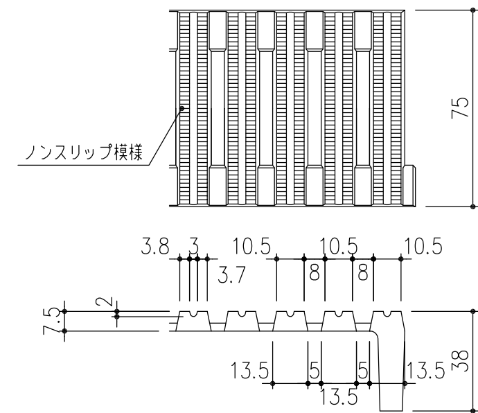
ノンスリップ詳細図 S=1/2
