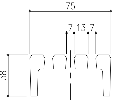
スレンダー側溝蓋 詳細図 S=1/2
