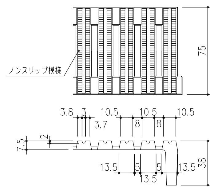
ノンスリップ詳細図 S=1/2
