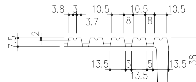
ノンスリップ詳細図 S=1/2
