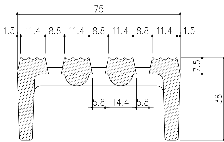
部分詳細図 S=1/1
