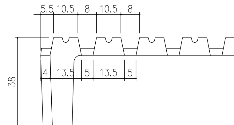
断面詳細図 S=1/1
