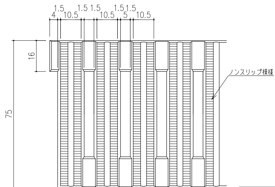
平面詳細図 S=1/1
