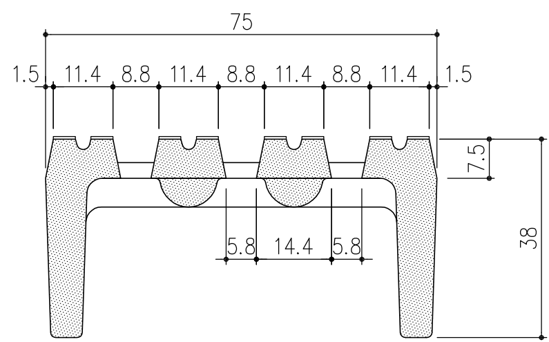
部分詳細図 S=1/1
