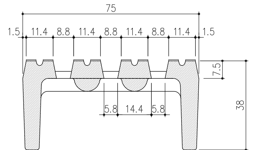
部分詳細図 S=1/1
