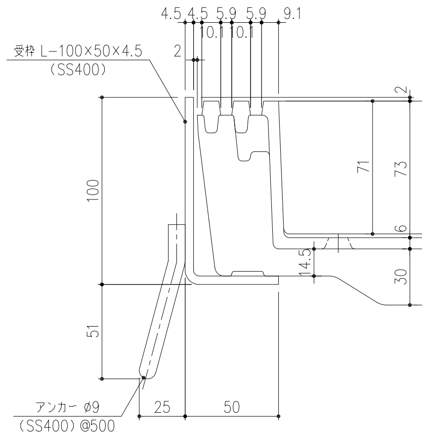
A部 詳細図 S=1/2
