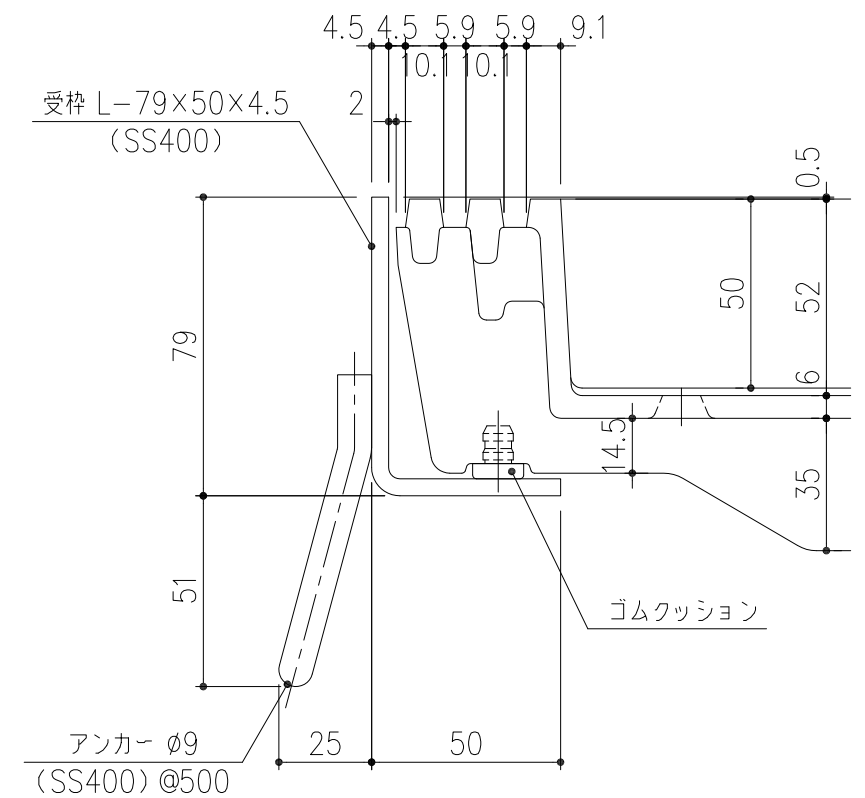
A部 詳細図 S=1/2
