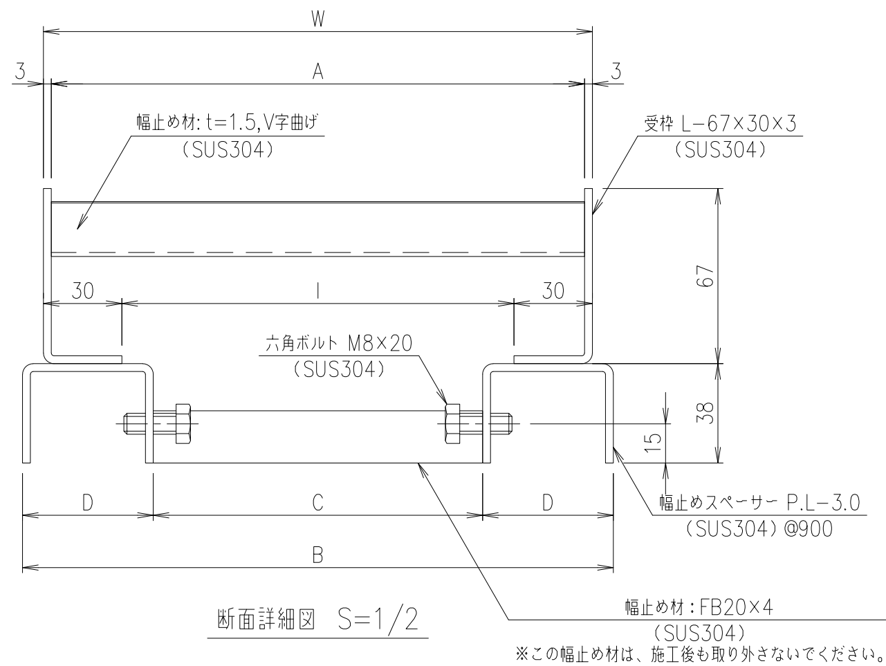
U字溝呼び 記 号 質量 kg/組 W A B C D \ell 150 210 204 226 126 50 150 10.4 180 260 254 266 166 60 200 10.6 240 310 304 346 212 67 250 10.8 300 360 354 416 282 67 300 11.2
