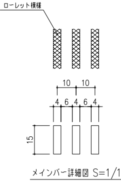
メインバー詳細図 S=1/1
