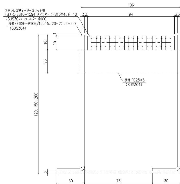
A-A 断面詳細図 S=1/1
