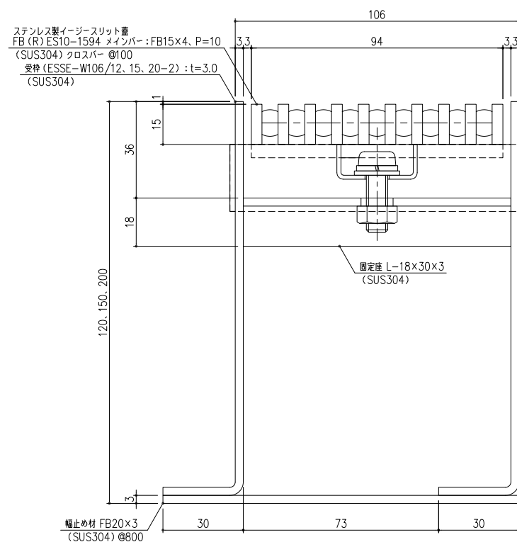
B-B 断面詳細図 S=1/1
