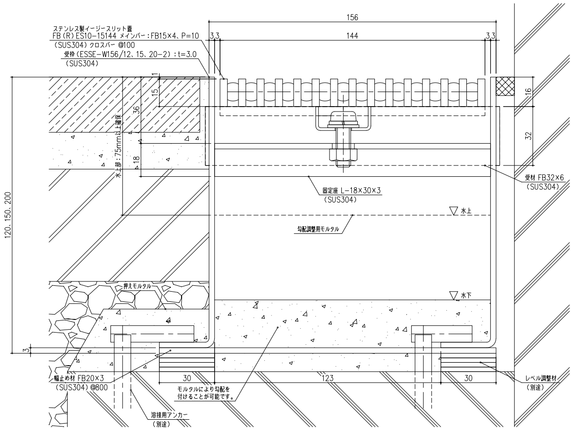
断面詳細図 S=1/1
