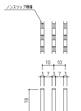
メンバー詳細図 S=1/1
