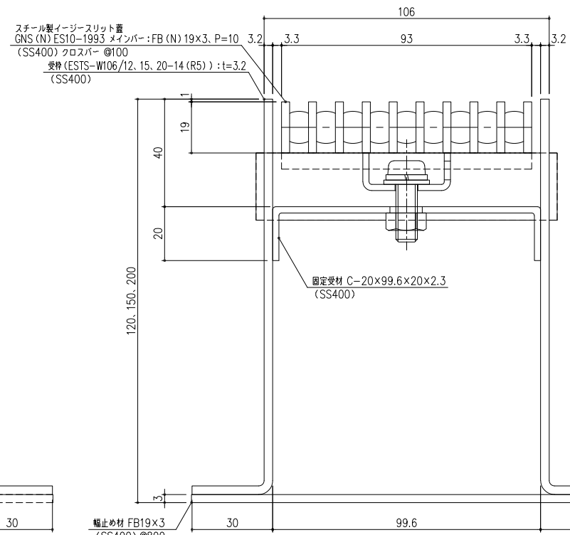
B-B 断面詳細図 S=1/1
