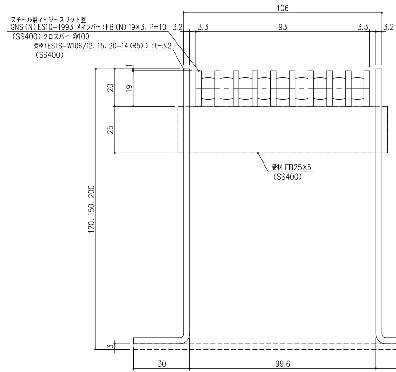
A-A 断面詳細図 S=1/1
