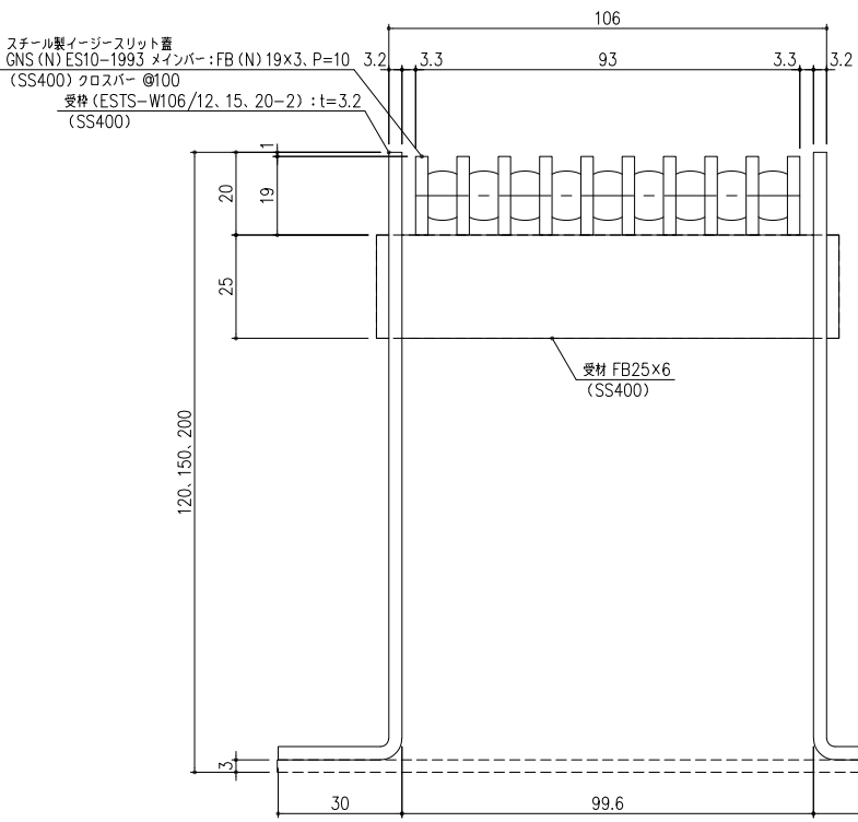
A-A 断面詳細図 S=1/1
