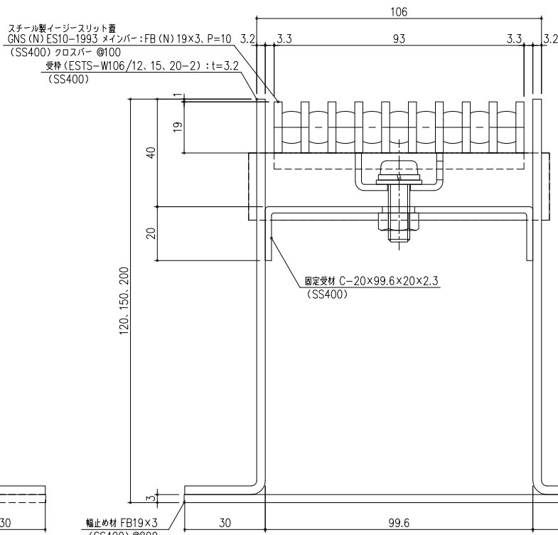
B-B 断面詳細図 S=1/1
