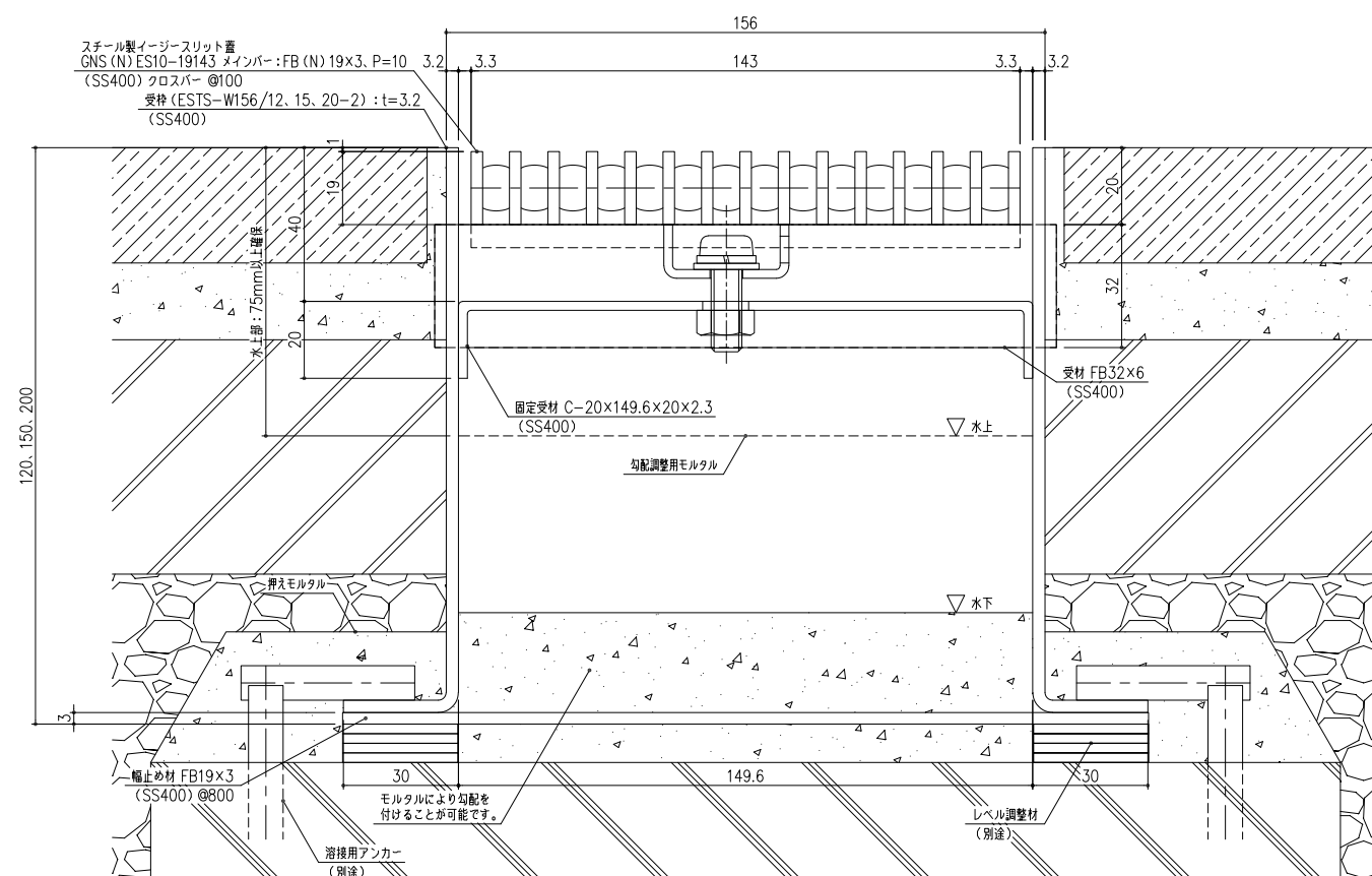
断面詳細図 S=1/1
