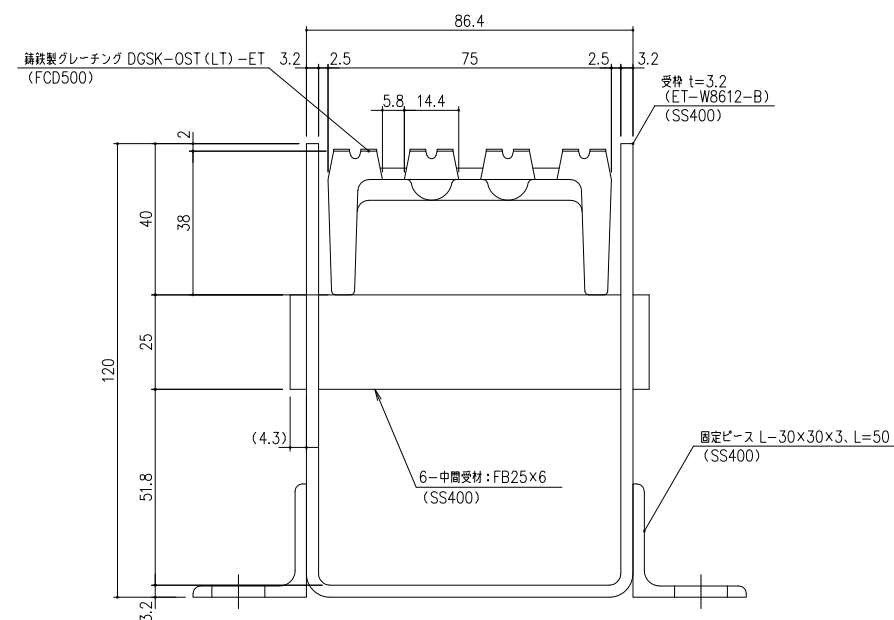
B-B 断面詳細図 S=1/1
