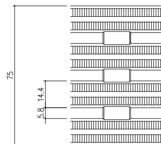
ET-DGSK-OST 平面詳細図 S=1/1
