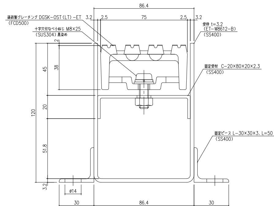
A-A 断面詳細図 S=1/1
