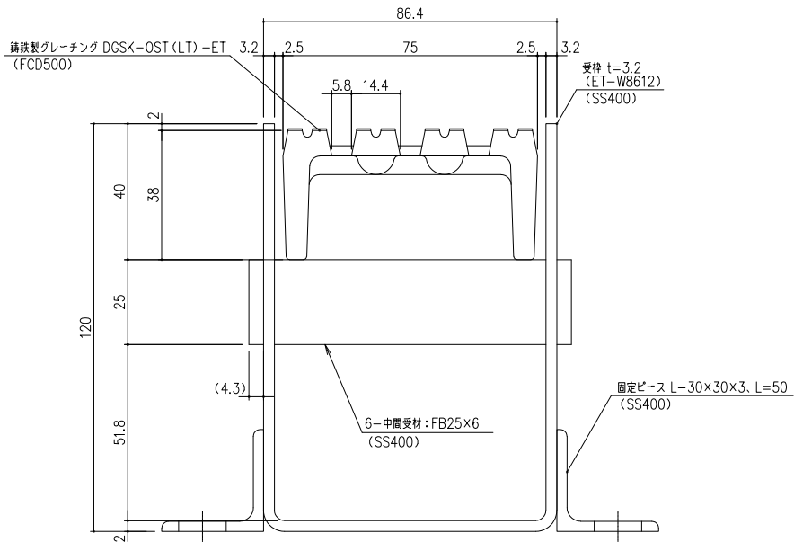
B-B 断面詳細図 S=1/1
