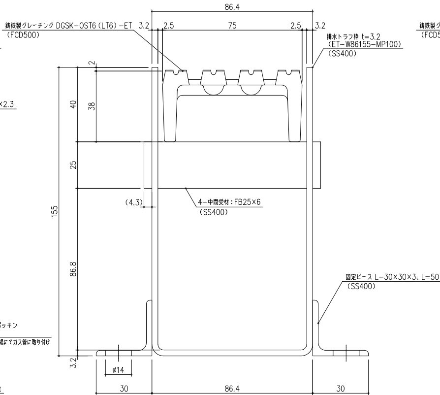
B-B 断面詳細図 S=1/1
