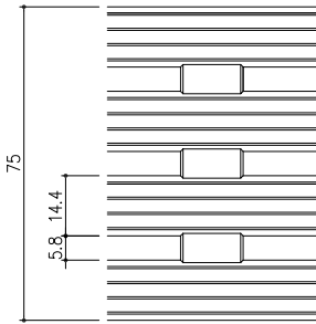
ET-DGSK-LT 平面詳細図 S=1/1
