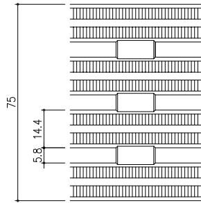
ET-DGSK-OST 平面詳細図 S=1/1
