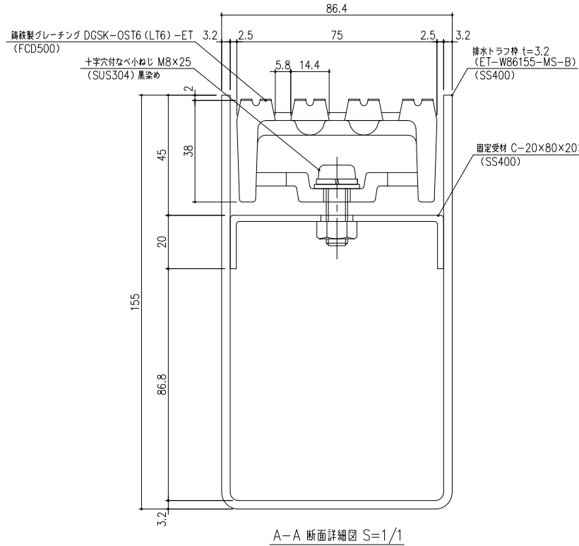
A-A 断面詳細図 S=1/1
