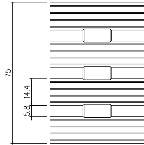
ET-DGSK-LT 平面詳細図 S=1/1
