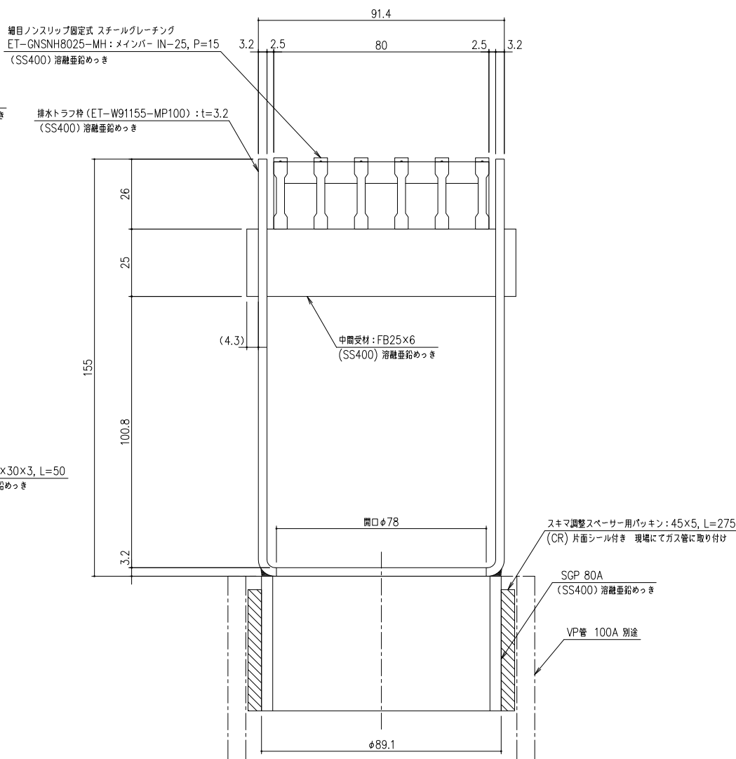
B-B 断面詳細図 S=1/1
