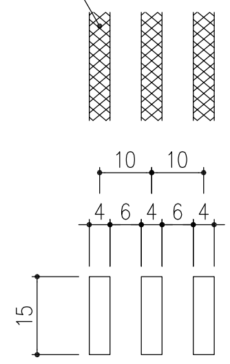
メインバー詳細図 S=1/1
