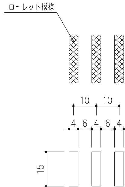
メンバー詳細図 S=1/1
