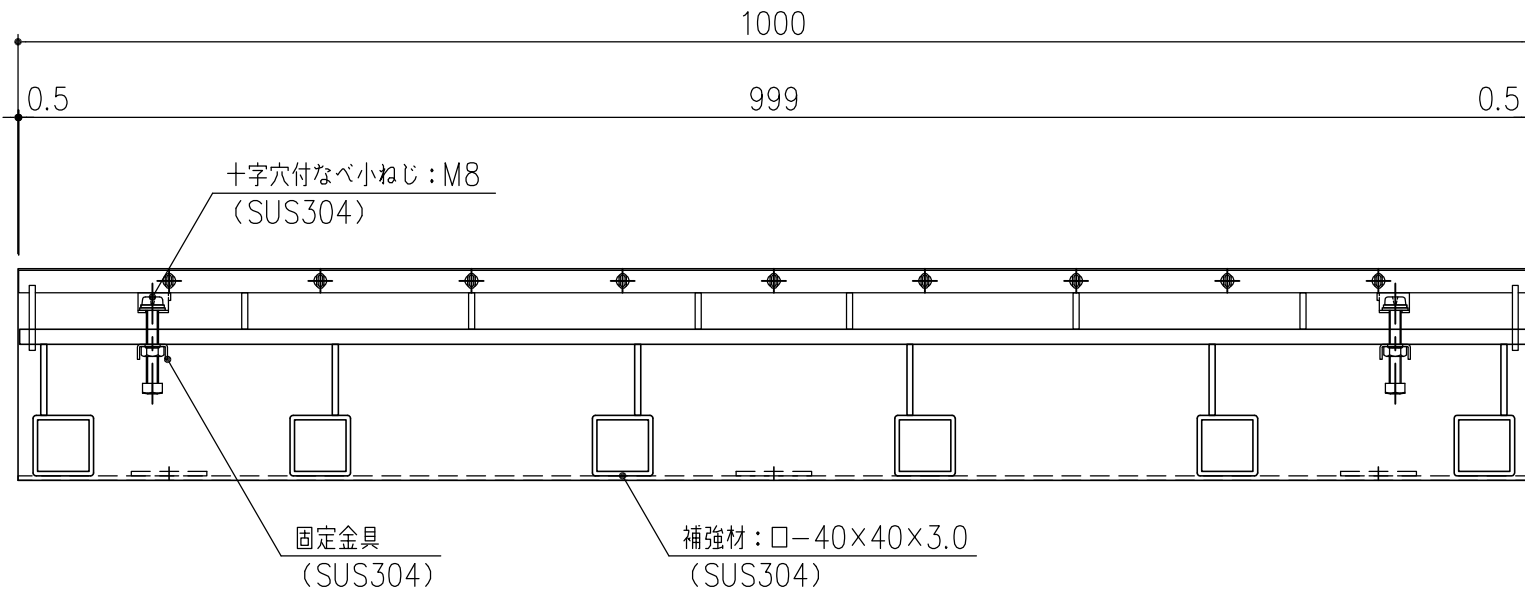
断面：A-A
