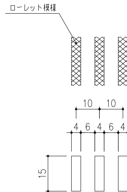
メインバー詳細図 S=1/1
