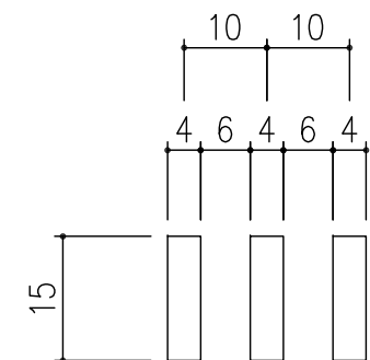
メンバーピッチ詳細図 S=1/1
