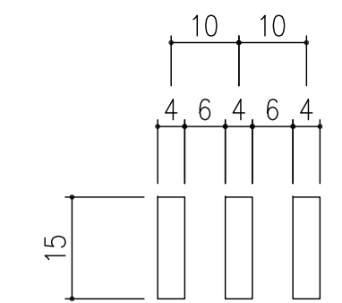
メインバーピッチ詳細図 S=1/1
