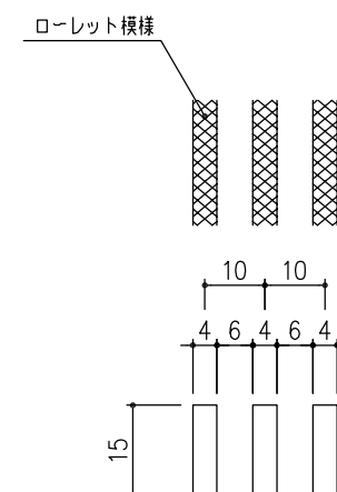
メンバー詳細図 S=1/1
