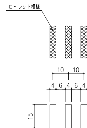
メンバー詳細図 S=1/1
