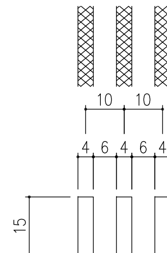
メンバーピッチ詳細図 S=1/1
