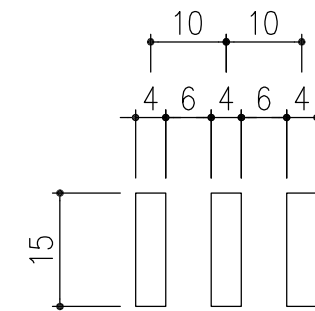
メインバー詳細図 S=1/1
