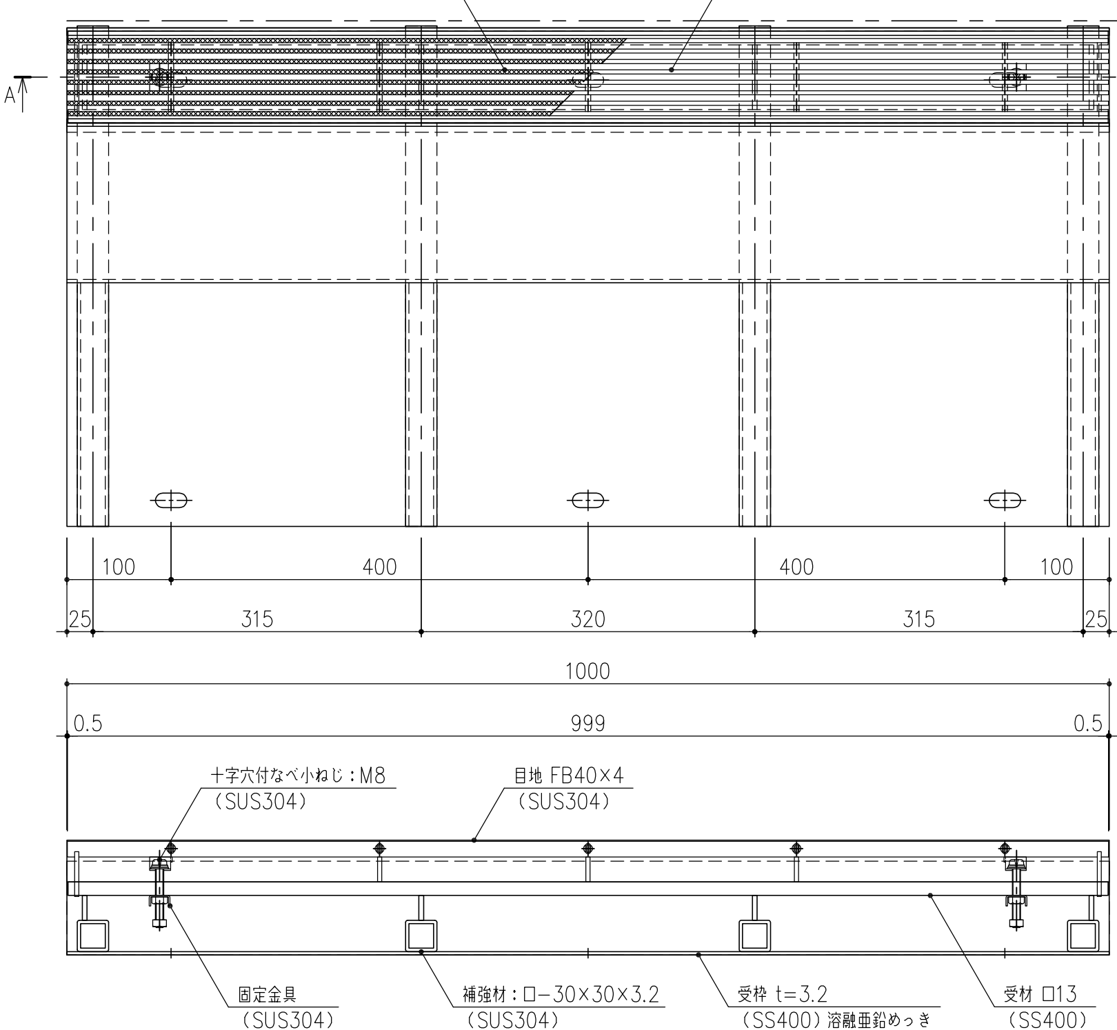
断面：A-A
