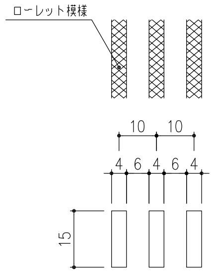
メインバー詳細図 S=1/1
