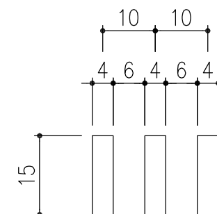
メンバー詳細図 S=1/1
