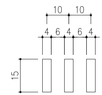
メインバー詳細図 S=1/1
