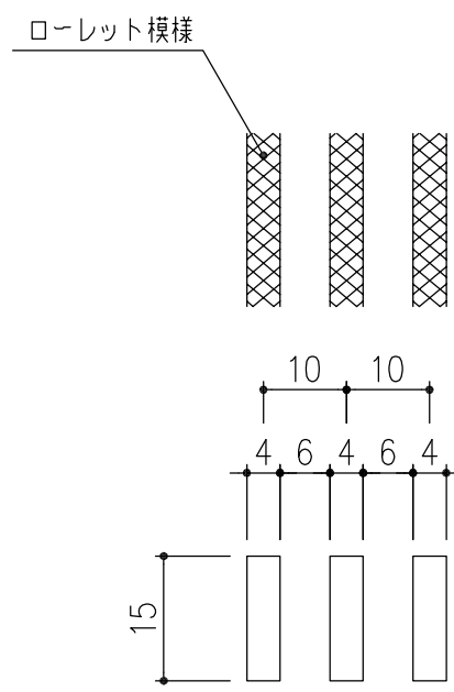
メインバー詳細図 S=1/1
