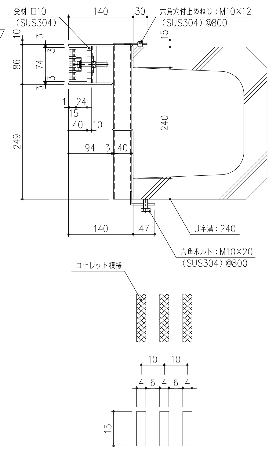
メインバー詳細図 S=1/1
