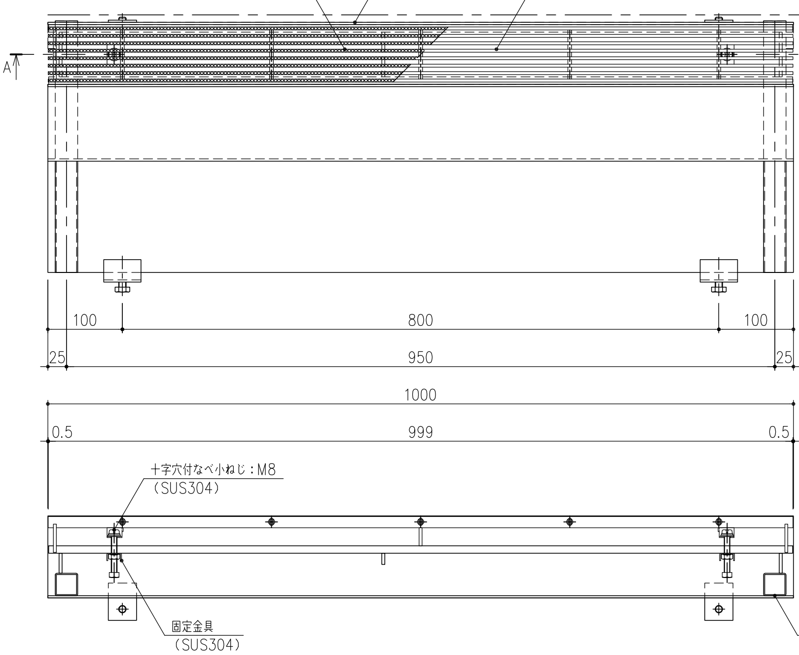
断面：A-A
