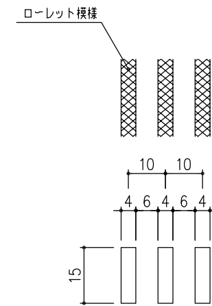
メンバー詳細図 S=1/1
